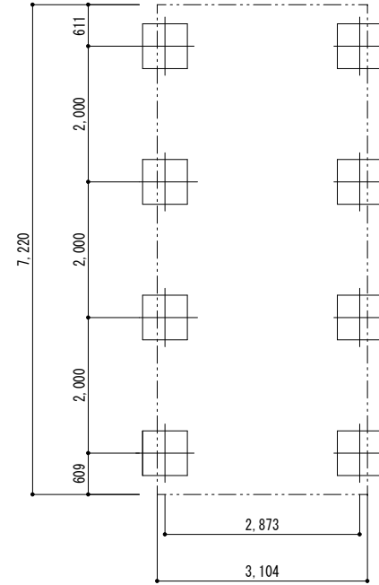
■ 基礎配置図
